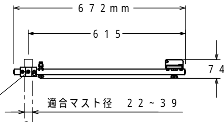
5 マスト固定金具
